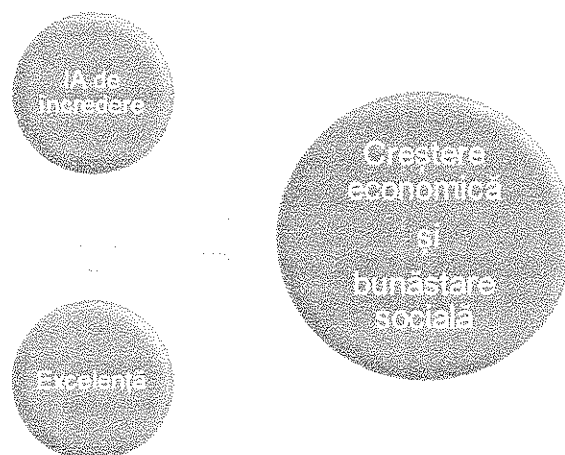
Figura 2.1. Viziunea SN-IA
